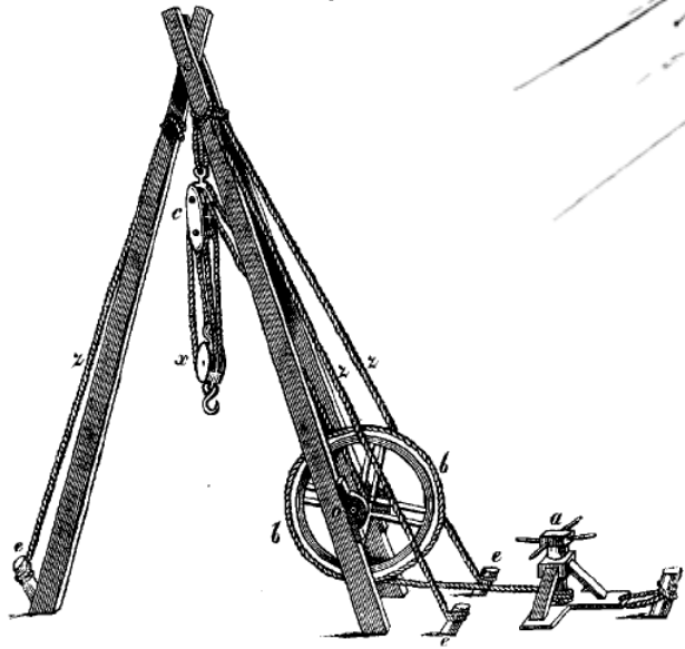
Machines de levage
