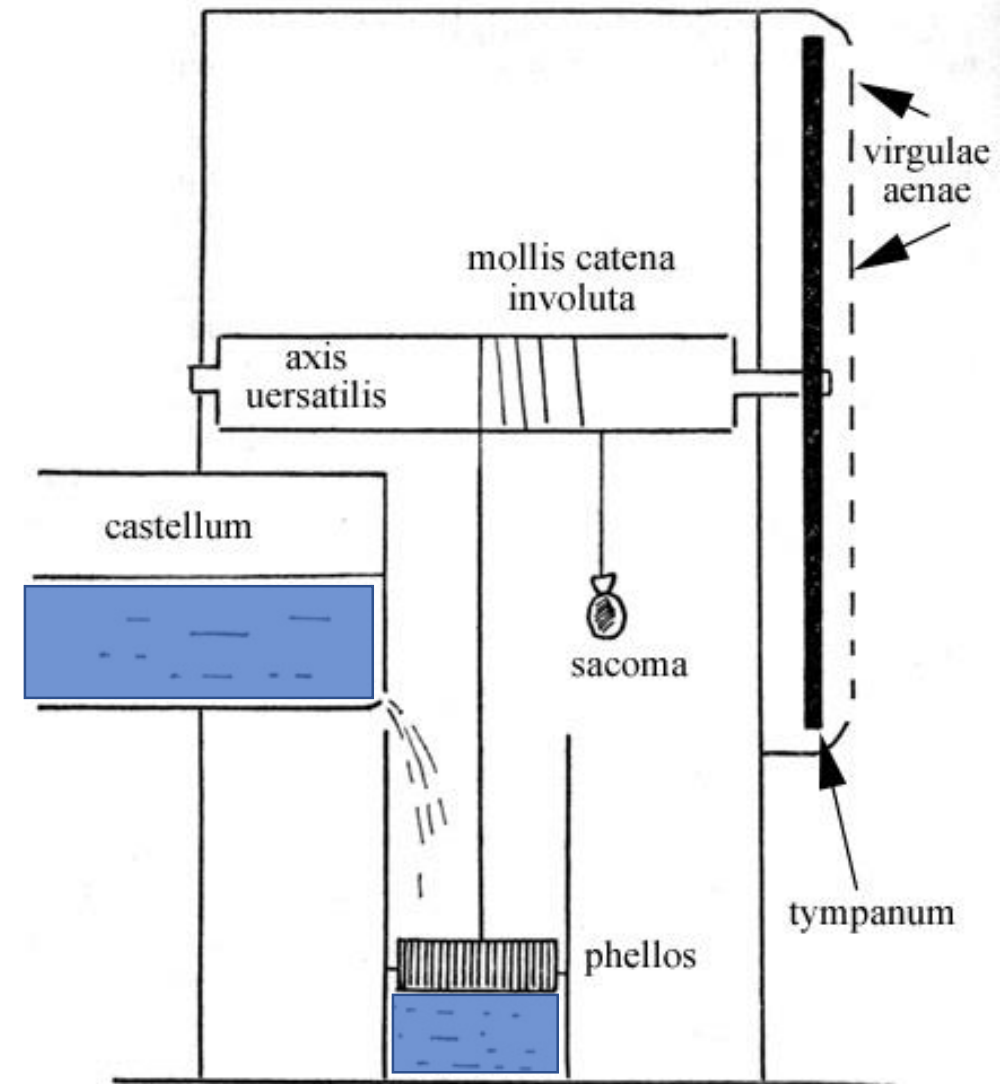
Horloge anaphorique de Vitruve. Cf. https://fr.wikipedia.org/wiki/Horloge_hydraulique_antique
